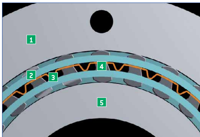
1 Bague extérieure 2 Cage 3 Ressort 4 Came 5 Bague intérieure
