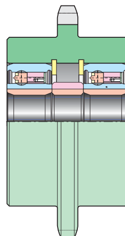
Montage intégré de roues libres CSK..P dans un pignon denté
