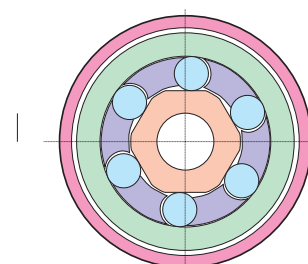
Embrayage à dépassement pour deux sens de rotation; changement de sens automatique
