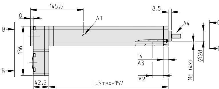
Bride C
